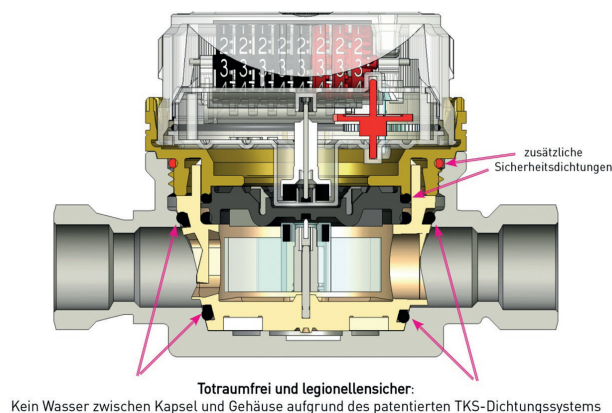
Patentiertes DELTAMESS-TKS-Kapselsystem
